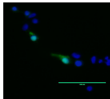
pEGFP-C1
